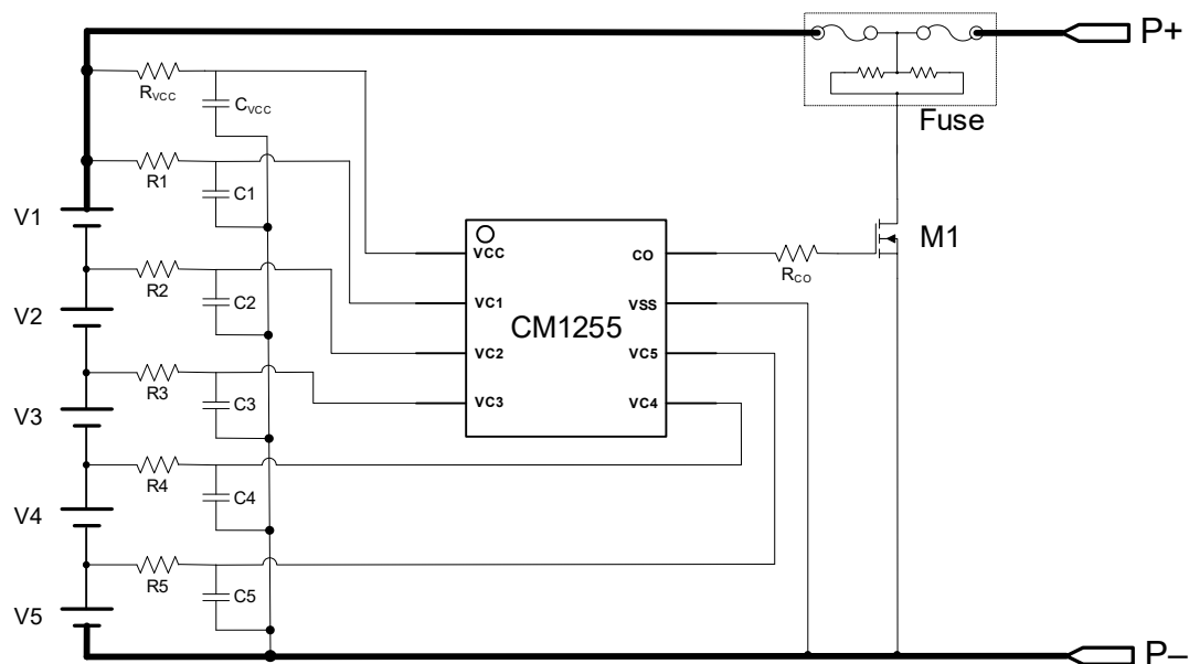
图 4 五串应用
