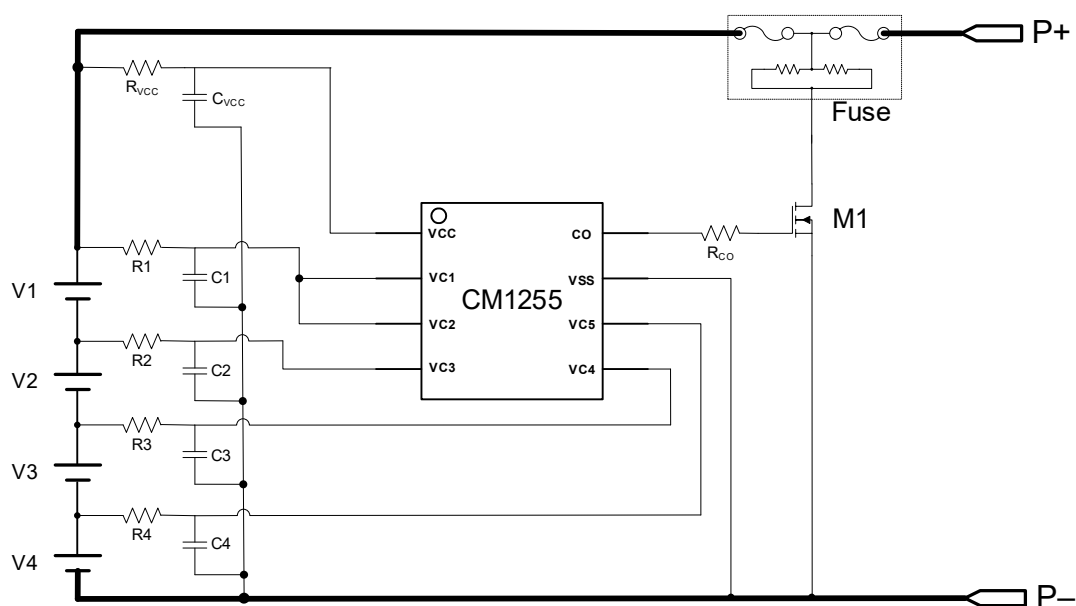
图 5 四串应用
