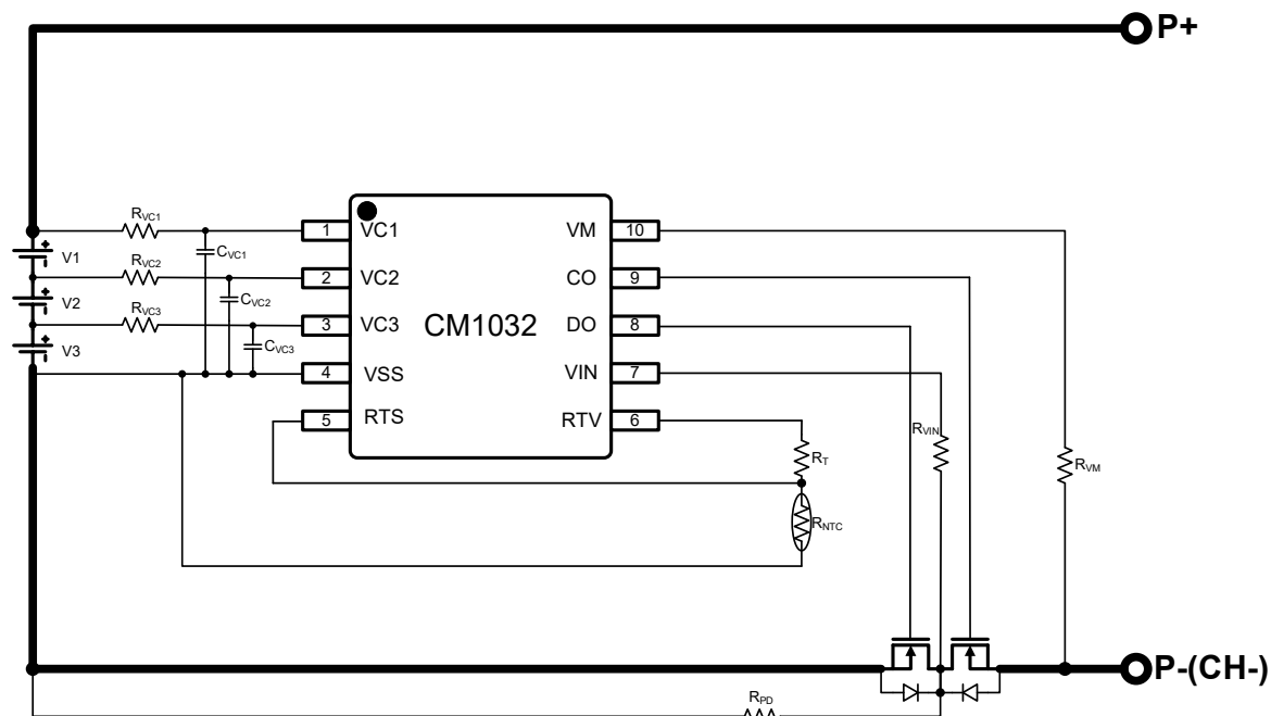
图 5 同口无检流电阻方案
