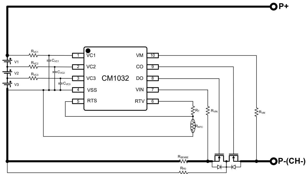
图 4 同口带检流电阻方案
