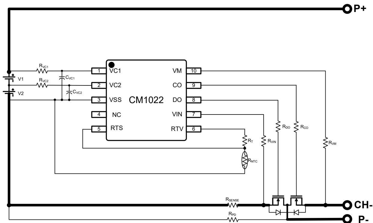
图 6 分口带检流电阻方案
