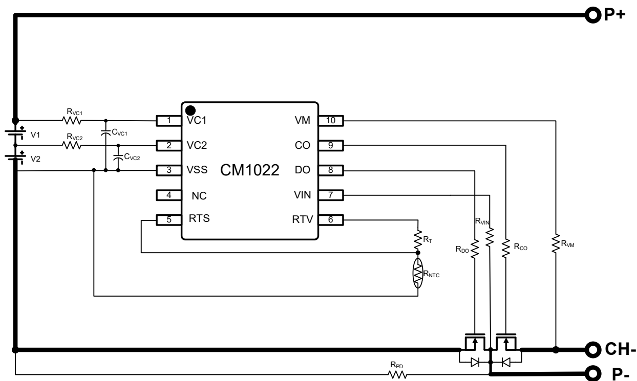
图 7 分口无检流电阻方案
