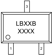
图 5 CM1823B
