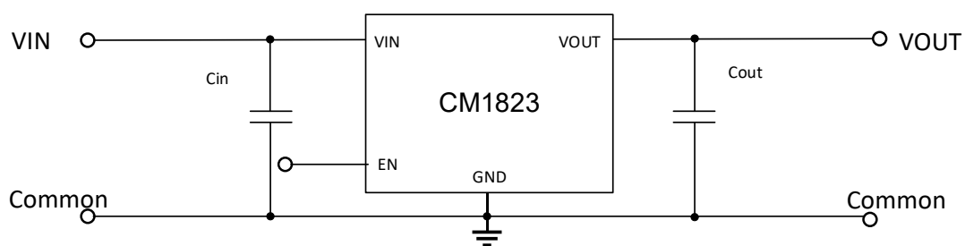
图 2 SOT23-5
