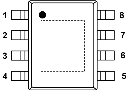
图 2 顶视图
