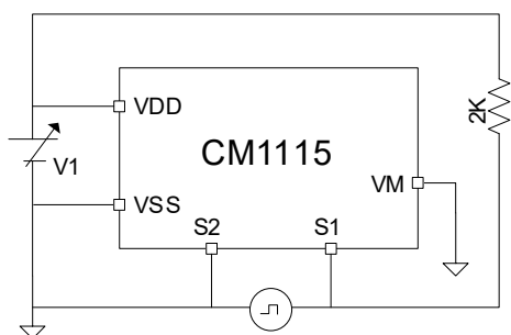
图 10 测试电路 3
