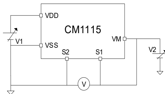
图 9 测试电路 2
