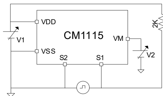
图 11 测试电路 4
