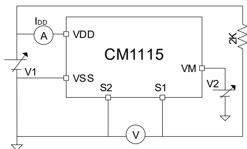
图 8 测试电路 1
