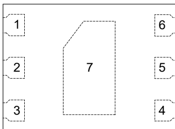
图 2 顶视图
