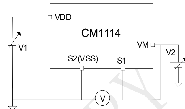
图 9 测试电路 2
