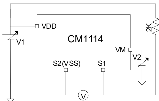
图 8 测试电路 1
