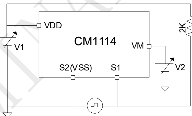
图 11 测试电路 4
