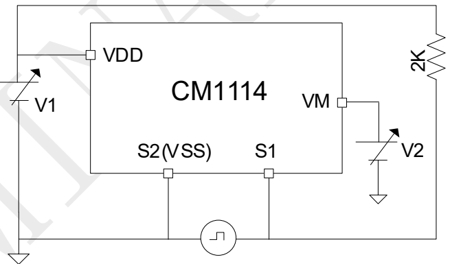
图 11 测试电路 4
