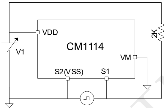
图 10 测试电路 3
