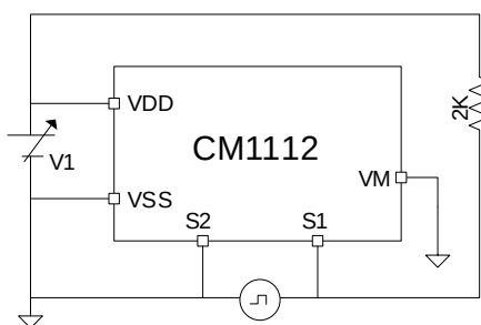
图 10 测试电路 3
