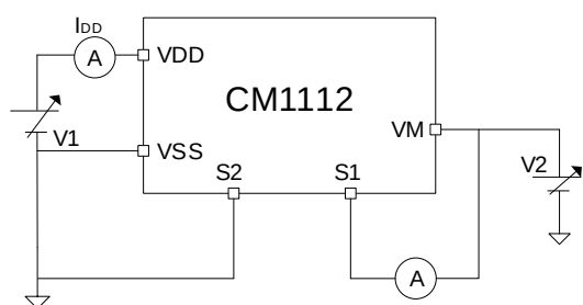
图 12 测试电路 5
