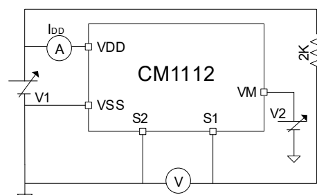
图 9 测试电路 2
