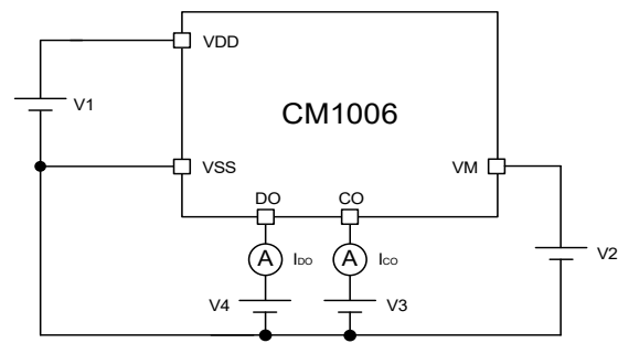
图 10 测试电路 4
