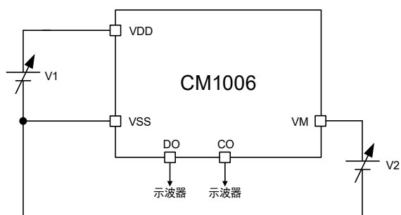
图 11 测试电路 5
