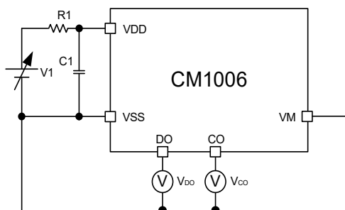
图 7 测试电路 1
