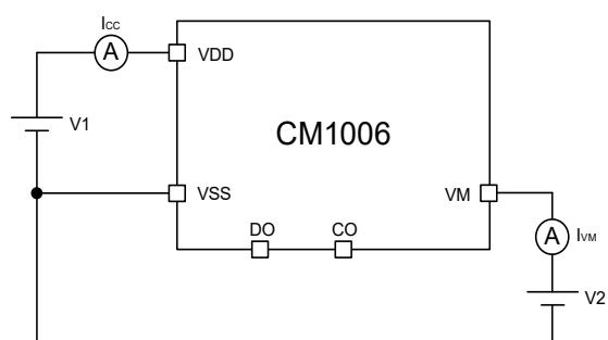
图 9 测试电路 3
