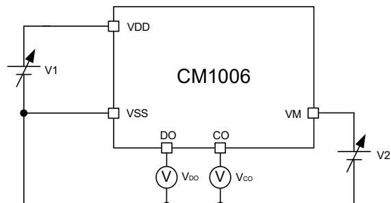
图 8 测试电路 2
