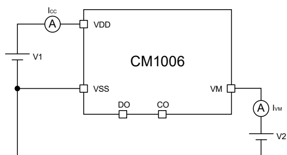
图 10 测试电路 3
