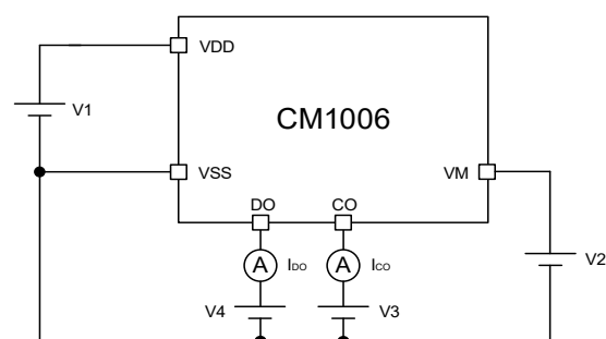
图 11 测试电路 4
