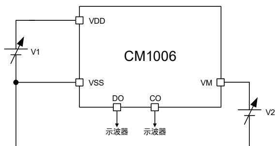
图 12 测试电路 5
