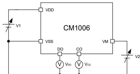
图 9 测试电路 2
