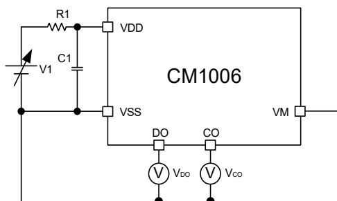
图 8 测试电路 1
