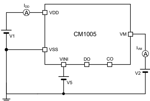
图 10 测试电路 3
