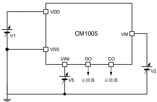
图 12 测试电路 5
