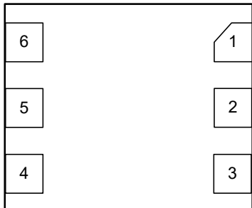
图 3 底视图
