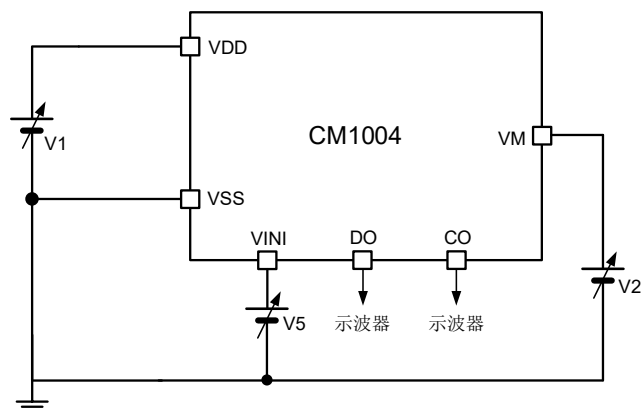
图 12 测试电路 5
