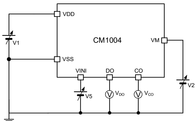
图 9 测试电路 2
