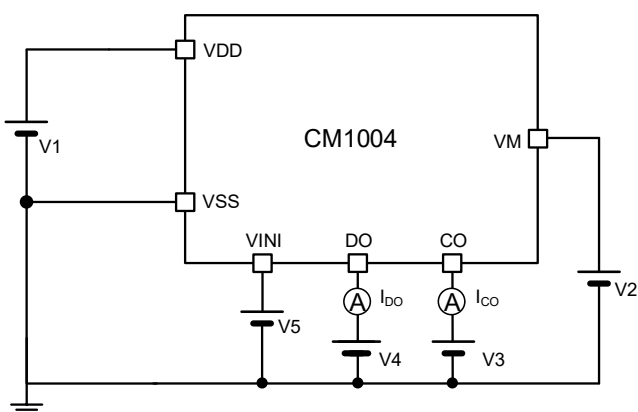
图 11 测试电路 4
