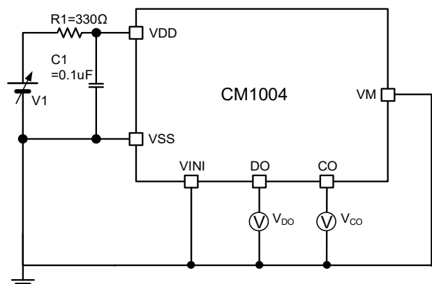
图 8 测试电路 1
