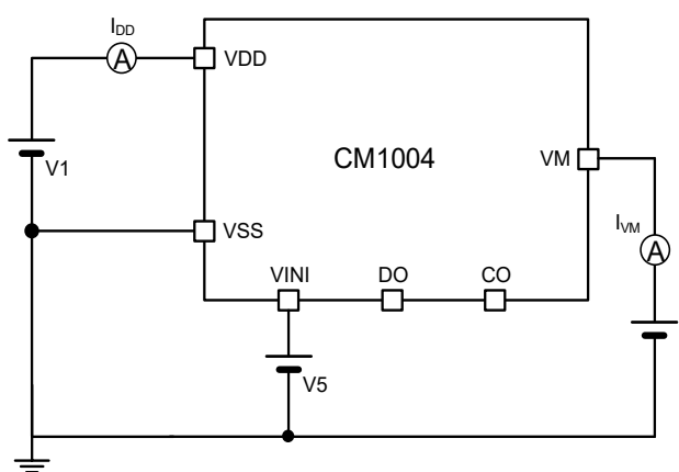
图 10 测试电路 3
