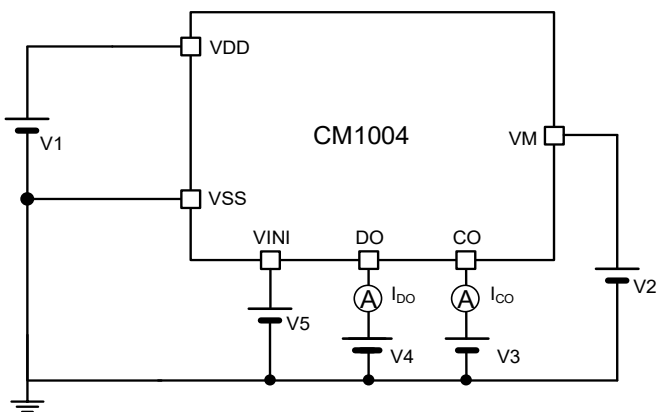
图 11 测试电路 4
