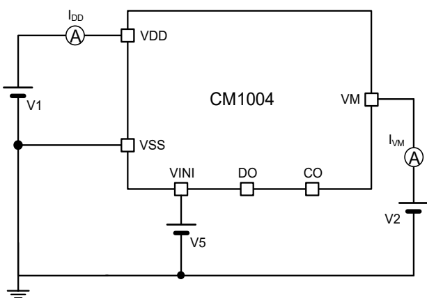
图 10 测试电路 3
