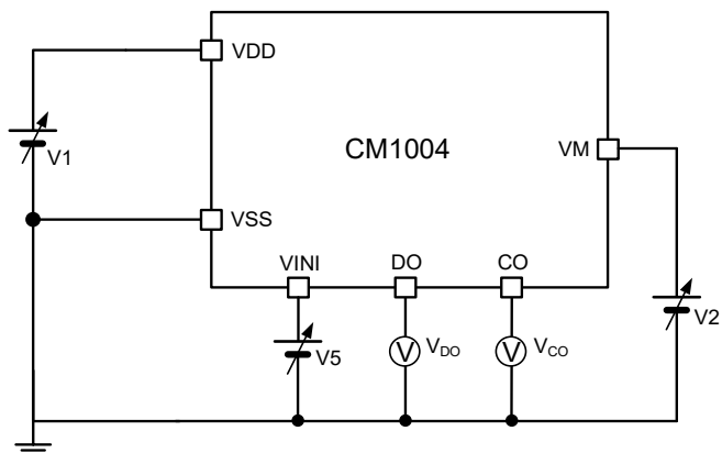
图 9 测试电路 2
