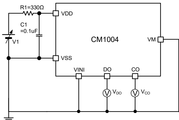
图 8 测试电路 1
