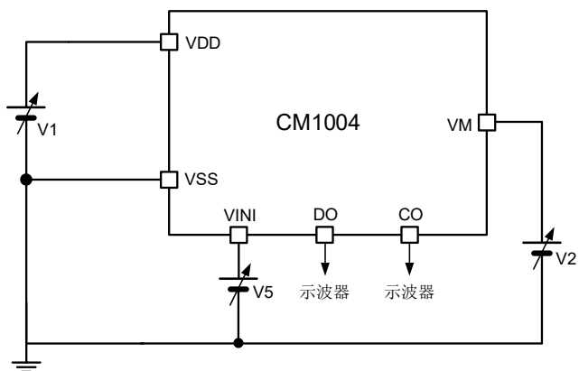
图 12 测试电路 5
