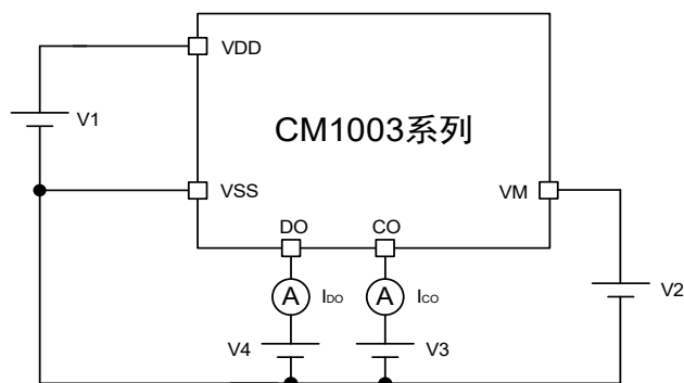
图 10 测试电路 4
