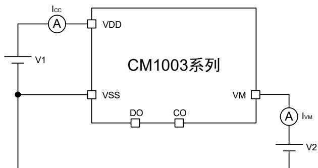
图 9 测试电路 3
