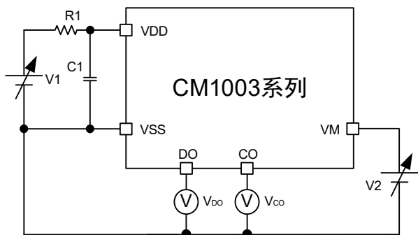
图 7 测试电路 1
