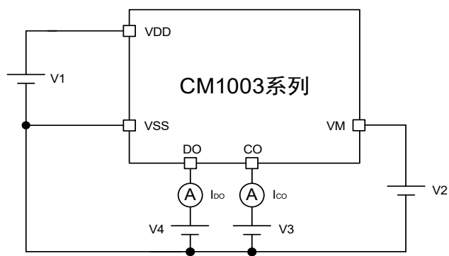
图 10 测试电路 4
