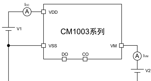
图 9 测试电路 3
