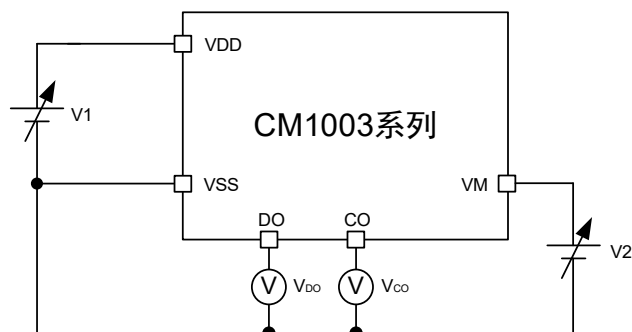
图 8 测试电路 2
