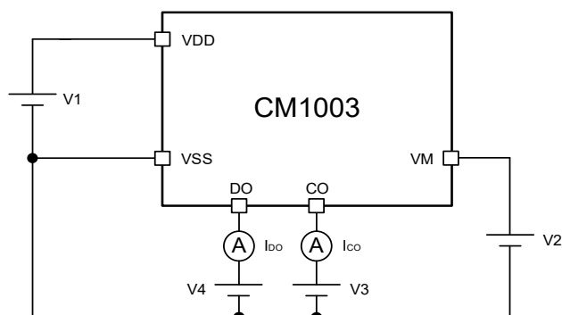
图 11 测试电路 4
