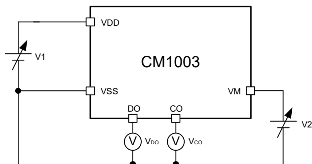
图 9 测试电路 2
