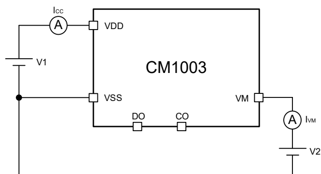
图 10 测试电路 3
