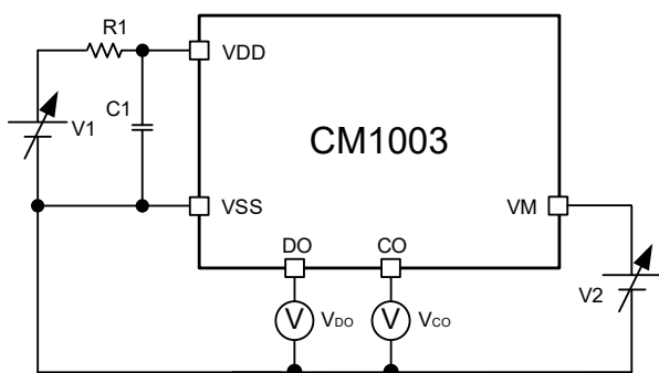
图 8 测试电路 1
