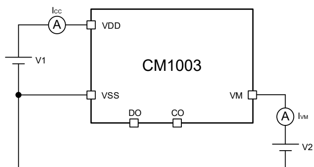
图 10 测试电路 3
