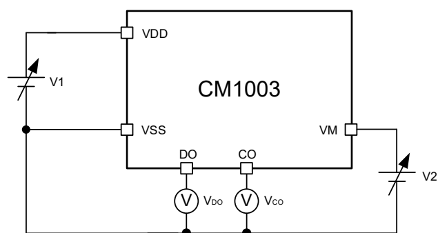
图 9 测试电路 2
