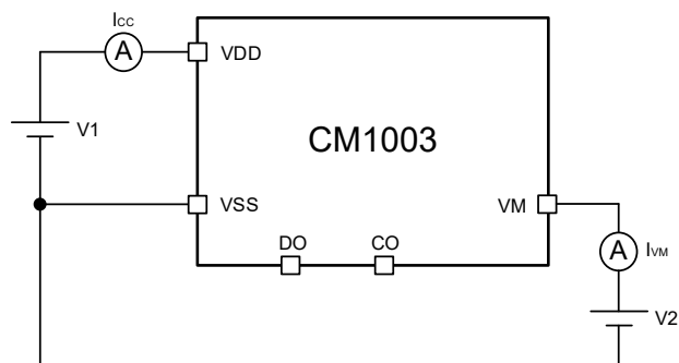
图 10 测试电路 3
