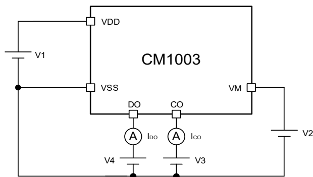
图 11 测试电路 4
