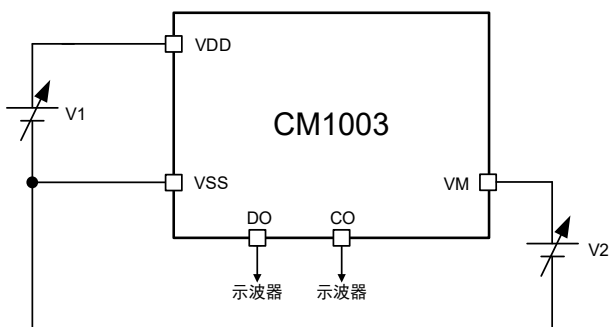
图 12 测试电路 5
