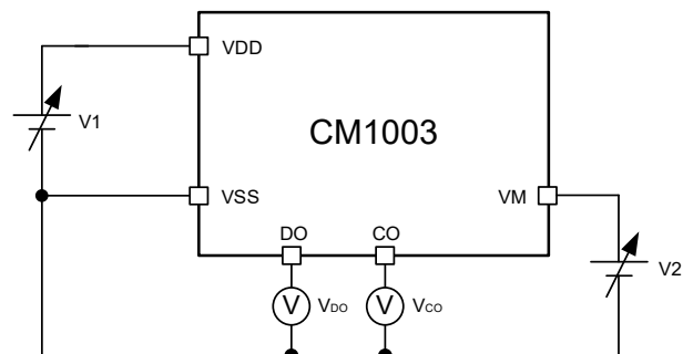
图 9 测试电路 2
