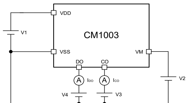
图 11 测试电路 4
