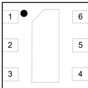
图 2 顶视图
