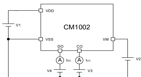
图 10 测试电路 4
