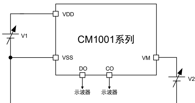
图 11 测试电路 5
