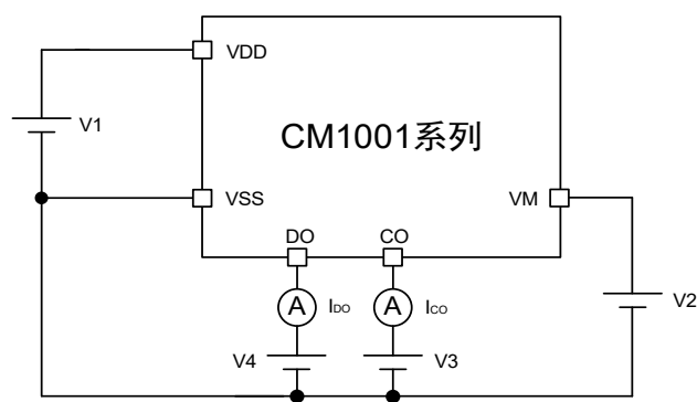
图 10 测试电路 4
