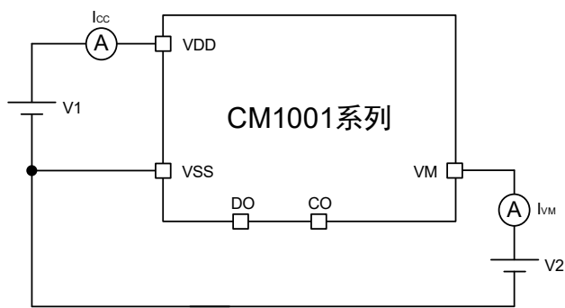
图 9 测试电路 3
